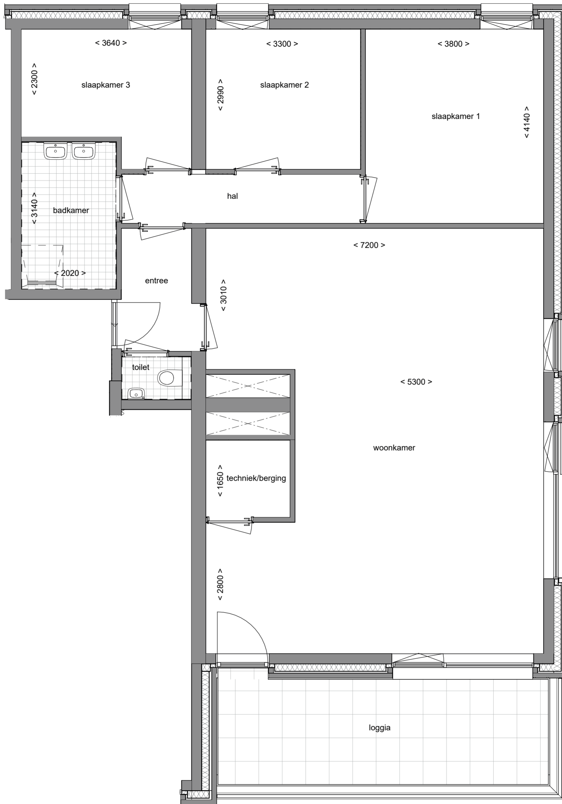
4-kamerappartement | derde verdieping bouwnummer 26
