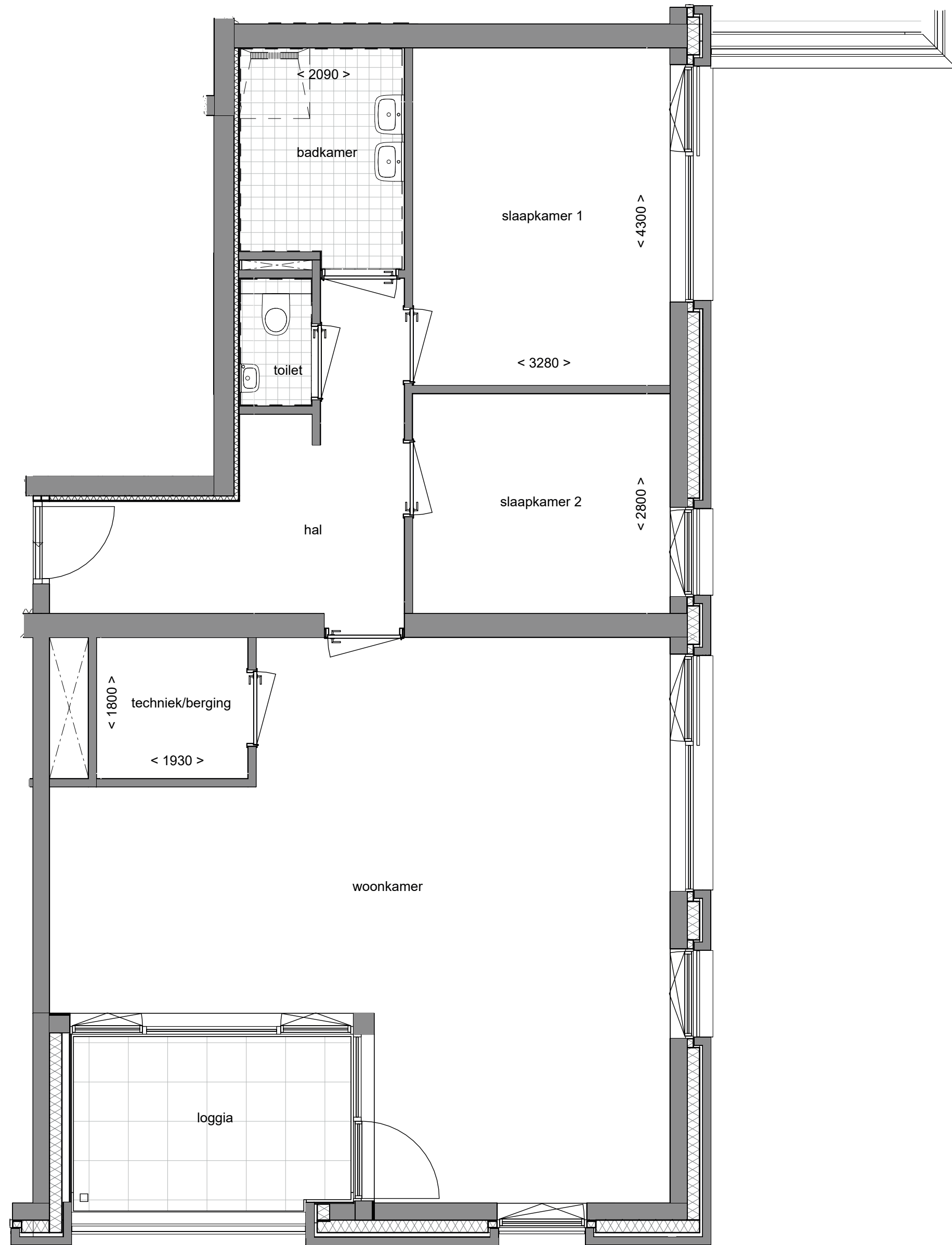
3-kamerappartement | eerste verdieping bouwnummer 15
